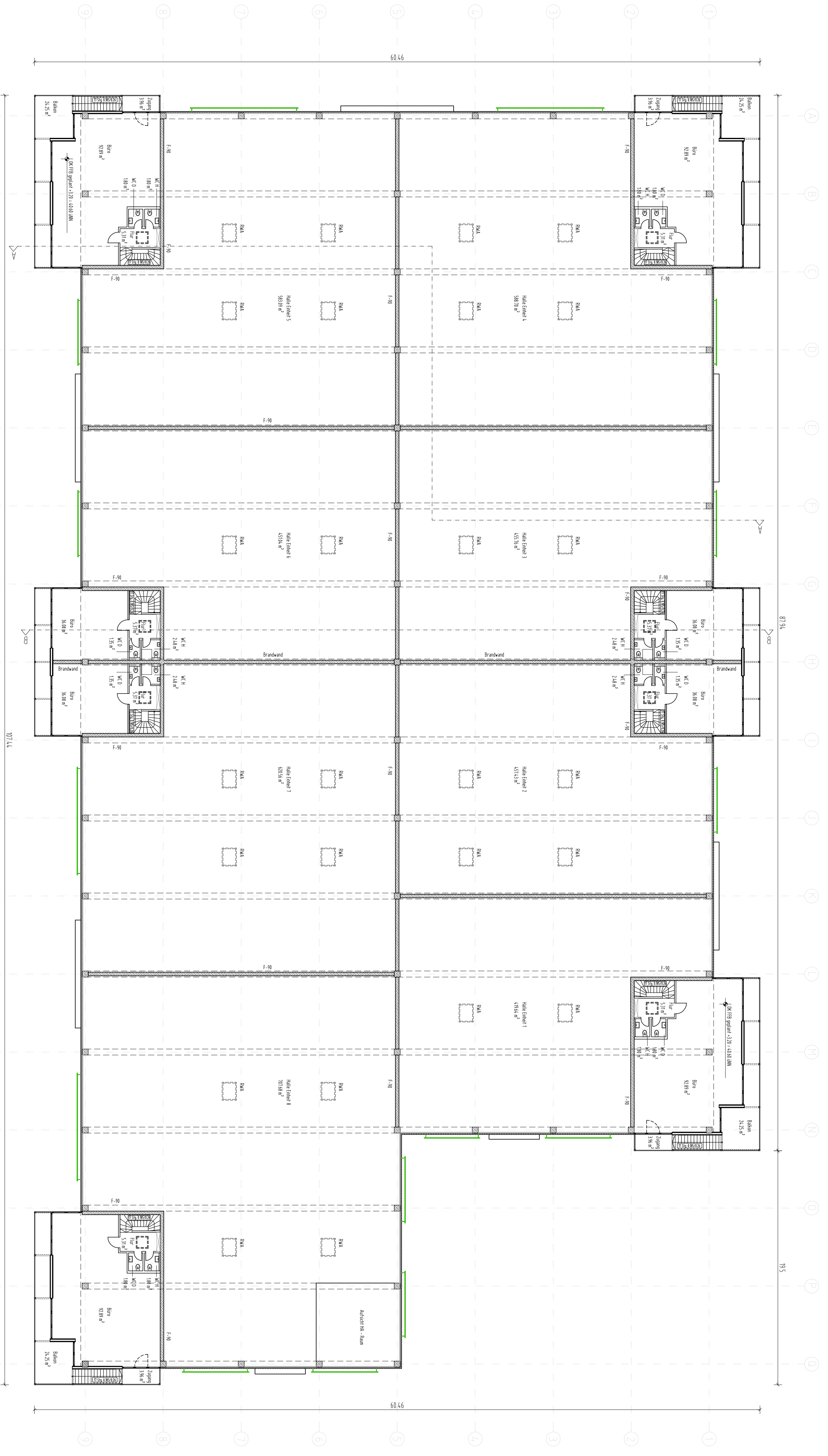
Grundriss Obergeschoss M. 1:200
