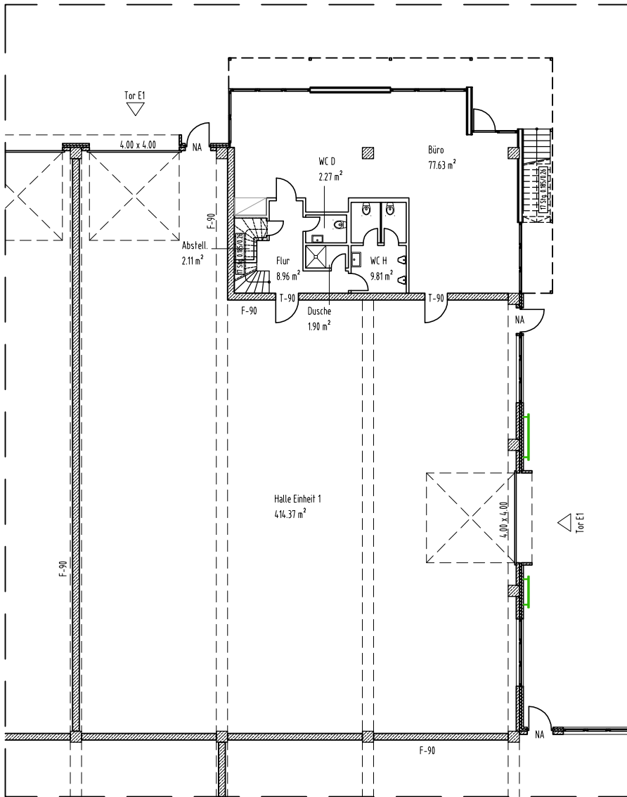
EINHEIT 1 Grundriss Erdgeschoss
