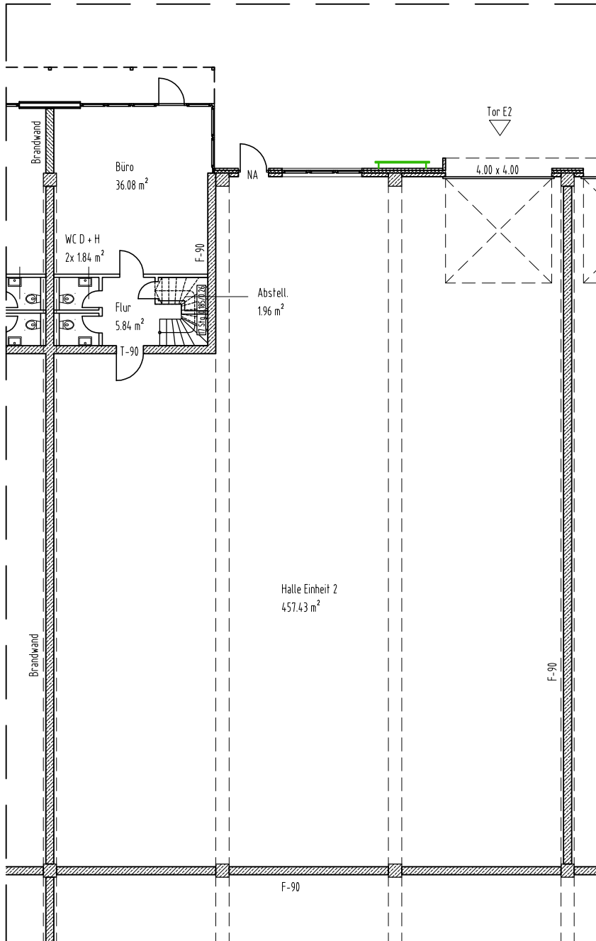
EINHEIT 2 Grundriss Erdgeschoss
