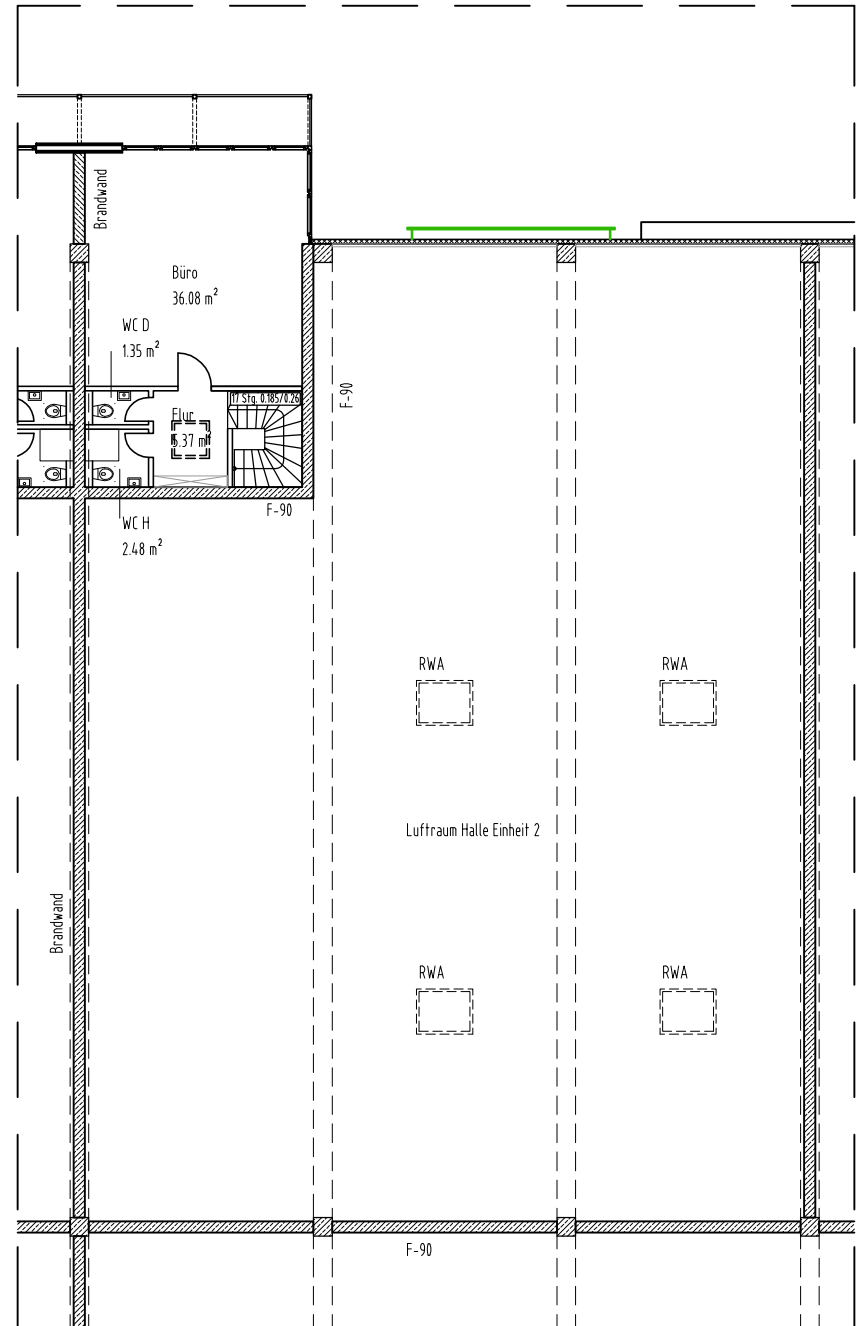
EINHEIT 2 Grundriss Obergeschoss
