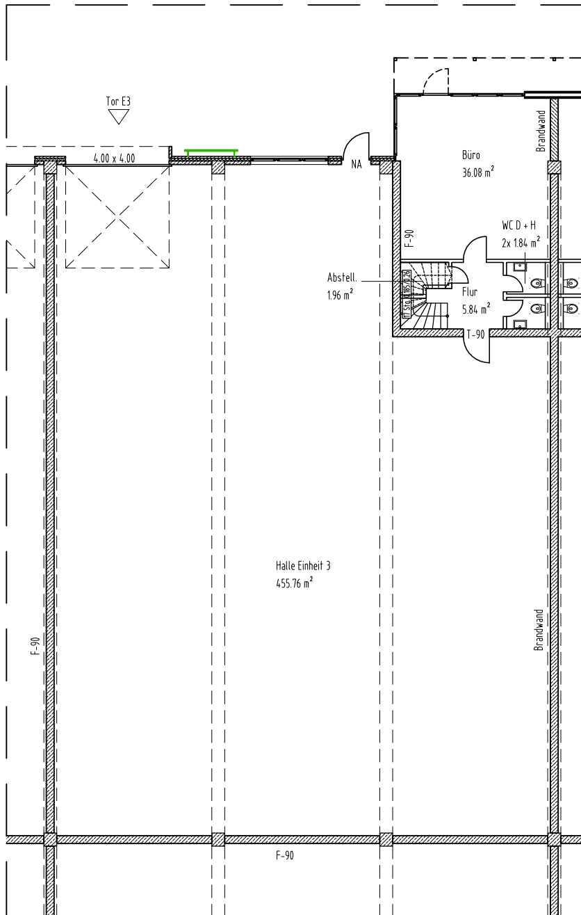
EINHEIT 3 Grundriss Erdgeschoss
