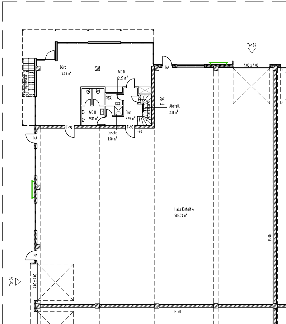
EINHEIT 4 Grundriss Erdgeschoss
