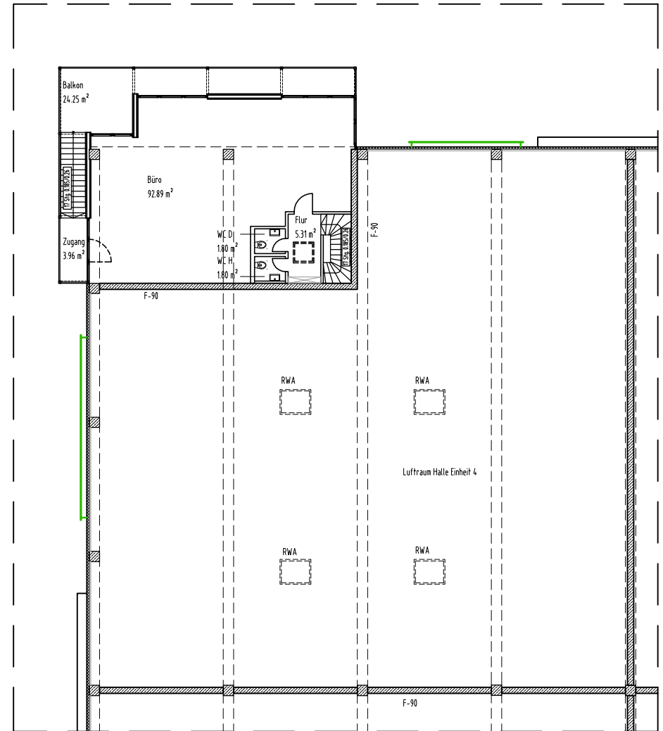
EINHEIT 4 Grundriss Obergeschoss
