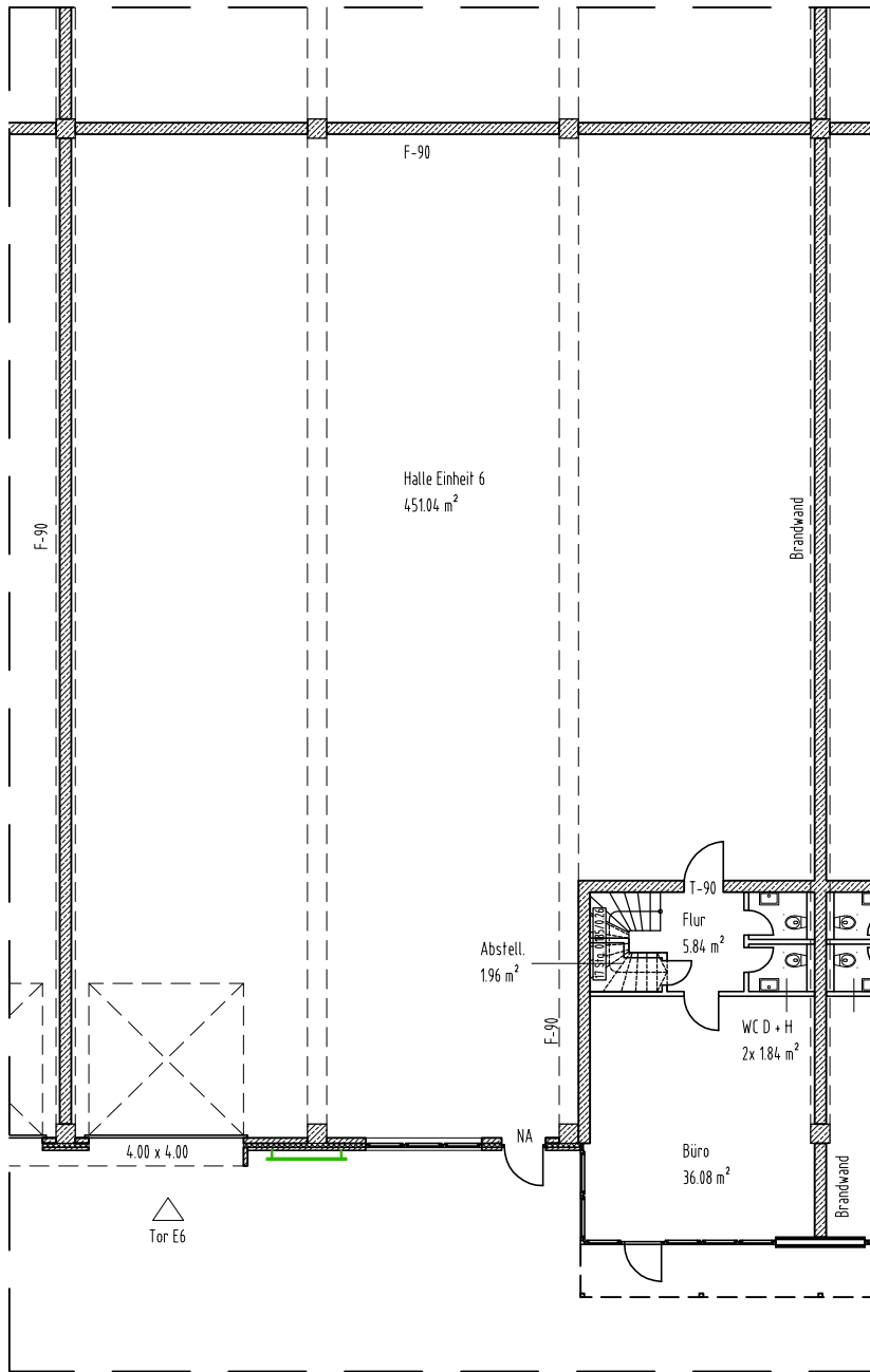
EINHEIT 6 Grundriss Erdgeschoss
