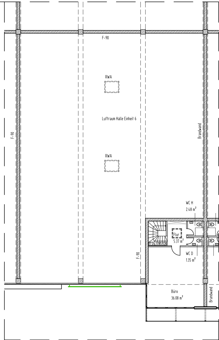
EINHEIT 6 Grundriss Obergeschoss
