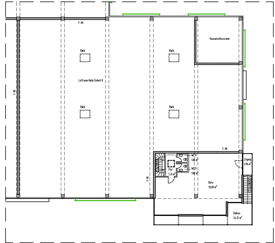
EINHEIT 8 Grundriss Obergeschoss
